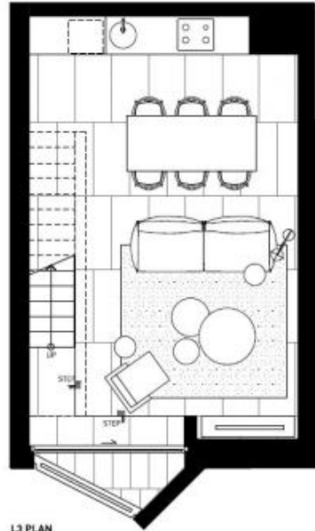
L3 PLAN
