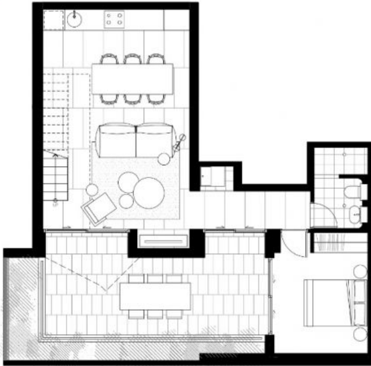
L1 PLAN
